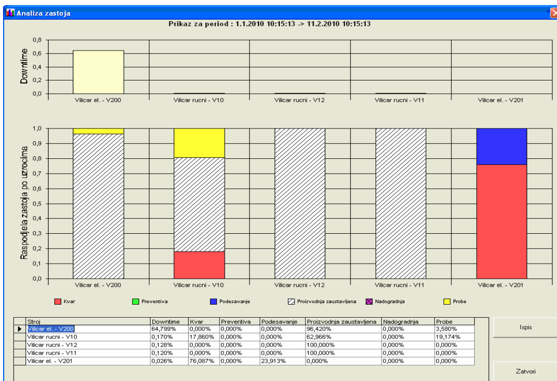
Izrada DOWNTIME izvještaja
